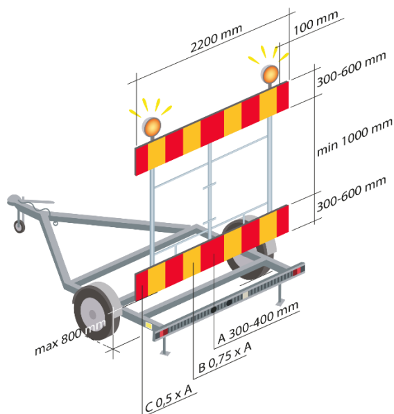
Illustration 9.5.1.1 Vägmarkesvagn
